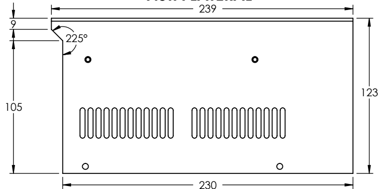
VISTA LATERAL
