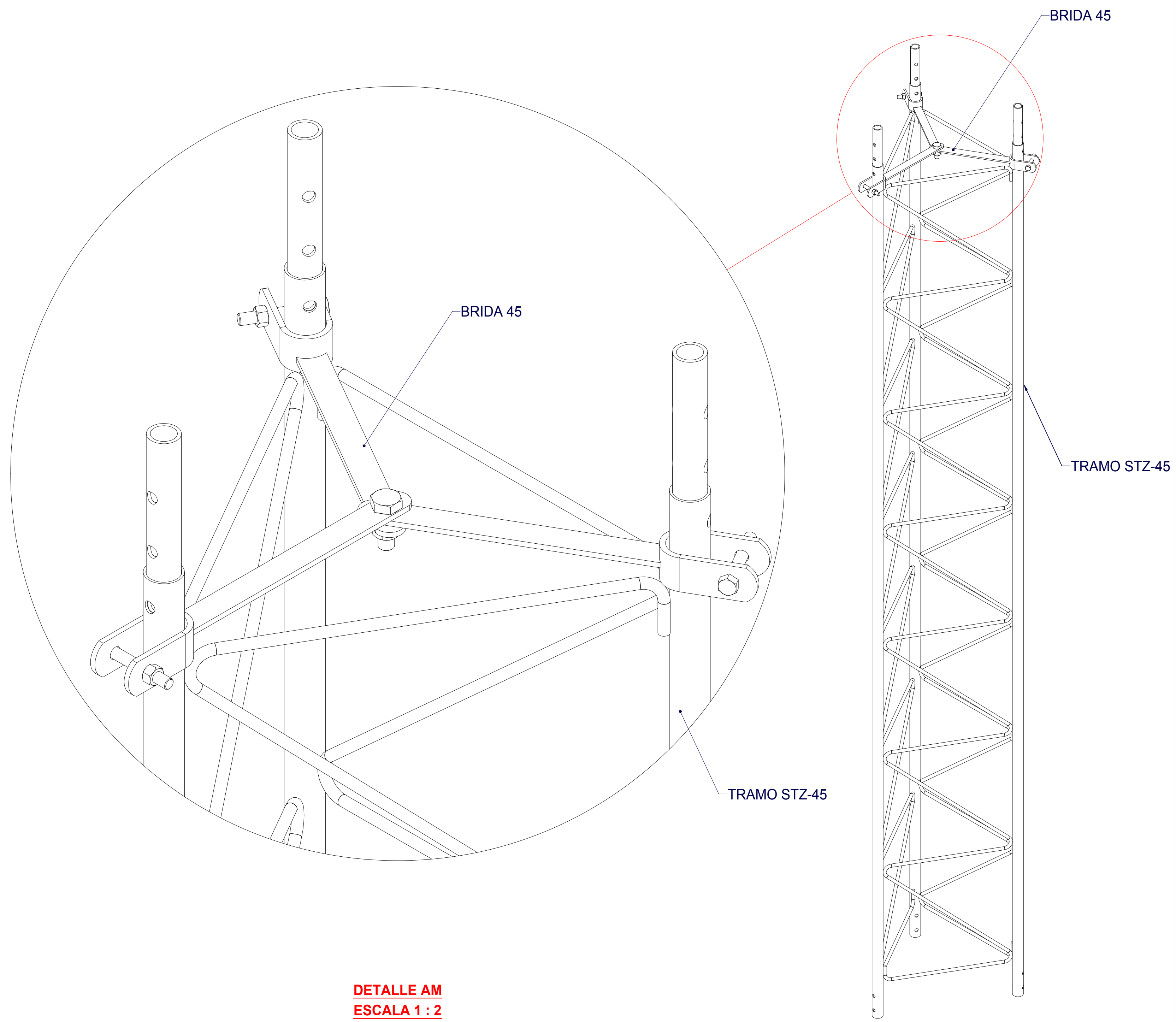
VISTA ISOMETRICA ENSAMBLAJE BRIDA 45 TRAMO STZ-45
