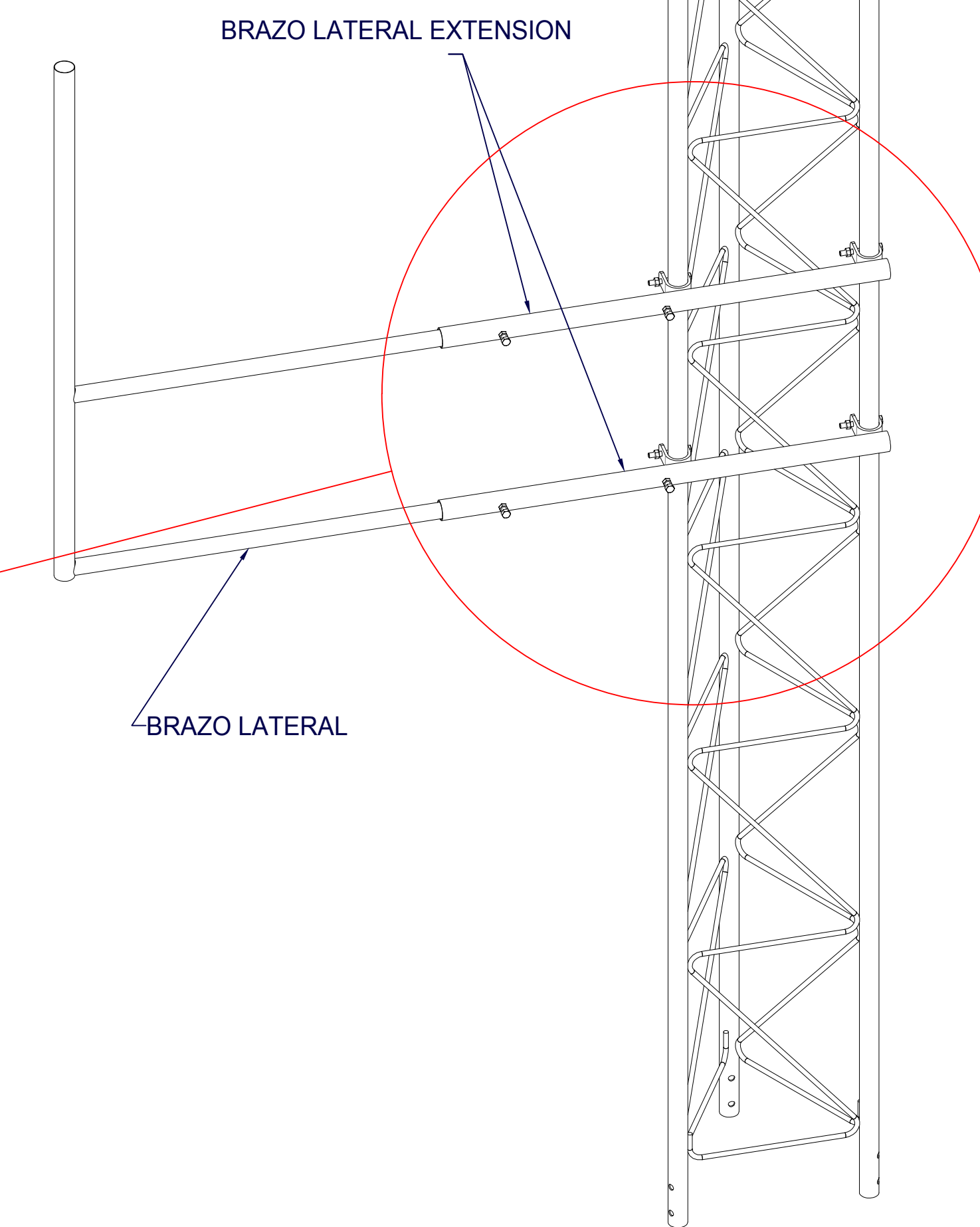
VISTA ISOMETRICA DE TRAMO STZ35 CON BRAZO LATERAL BLF Y BRAZO LATERAL EXTENSION SBL35
