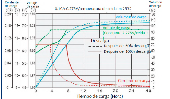
Curva característica de carga cíclica (25 °C/77 °F)
