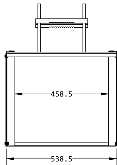
Vista superior. Medidas internas
