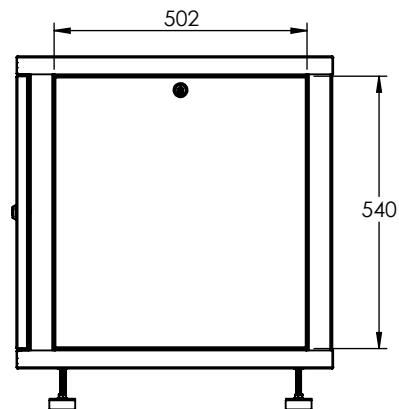
VISTA LATERAL
