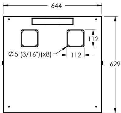
VISTA SUPERIOR
