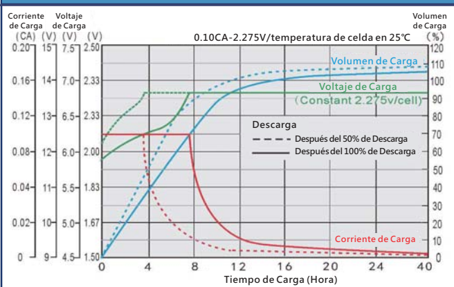
Curva característica de carga en flotante (25°C/77°F)
