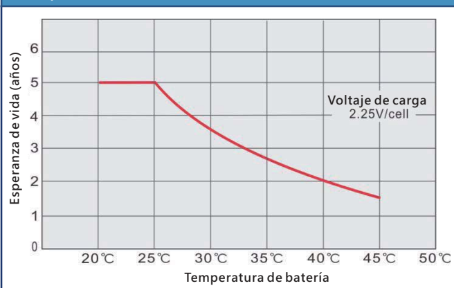
Temperatura vs Vida en flotación
