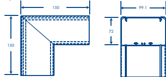
Esquinero exterior
