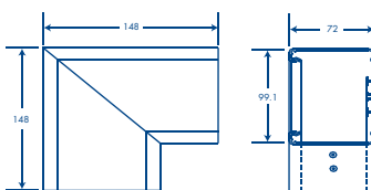
Sección L
