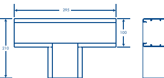
Sección T
