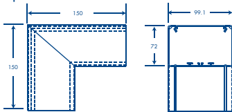
Esquinero interior
