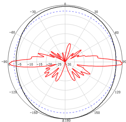
H-Pol @ 2450MHz
