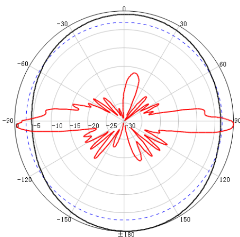
H-Pol @ 2450MHz
